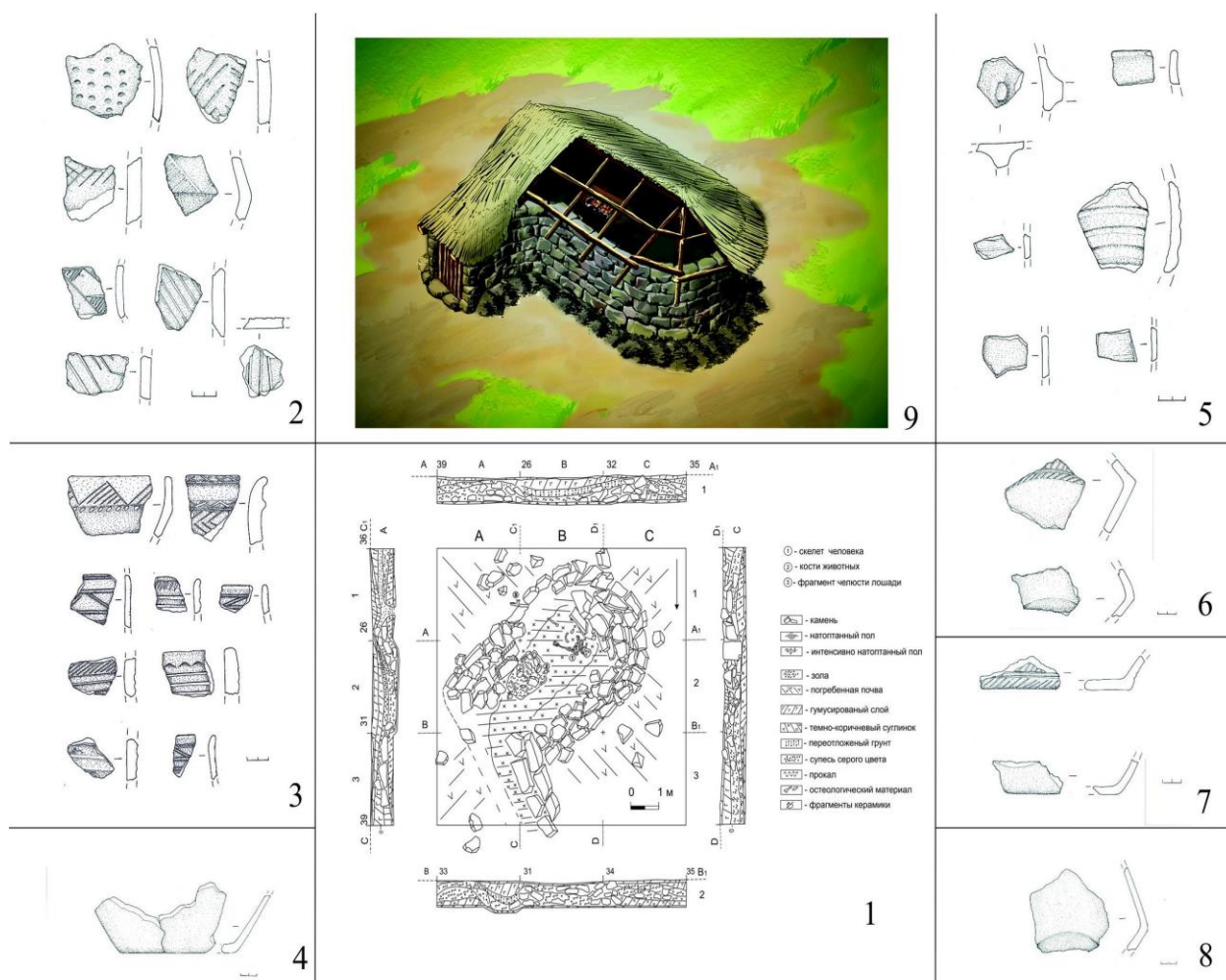
Рис. 3. Поселение Шагалаы II. Третий тип дома с каменными стенами. 1 – план и разрез жилища; 2-3 – фрагменты венчиков и стенок керамических сосудов; 5 – фрагменты импортной среднеазиатской станковой керамики; 4, 6-8 – фрагменты дна керамических сосудов, найденные возле очага; 9 – графическая реконструкция жилища № 6 с каменными стенами. Автор реконструкции Сакенов С.К., художник Меденко В.С.
